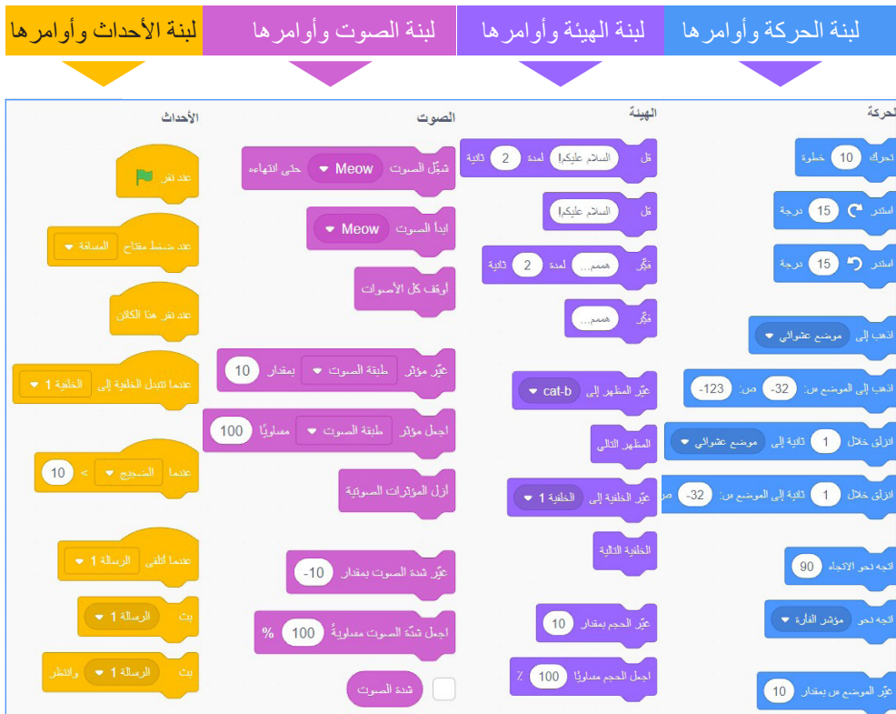
الشكل (١٦) بعض اللبنة في سكراتش
